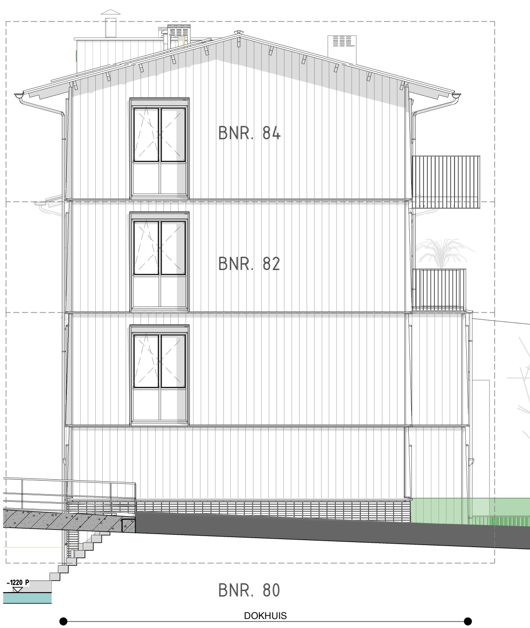
KOPGEVEL NOORD-OOST 1 : 100
