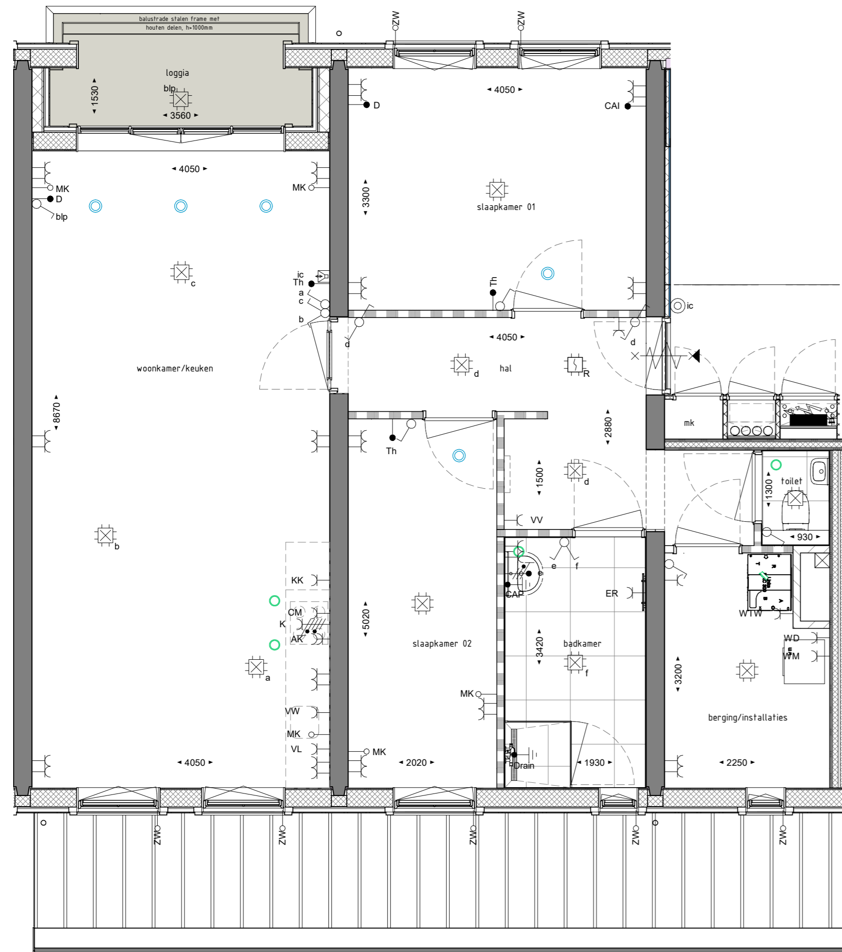
1E VERDIEPING
