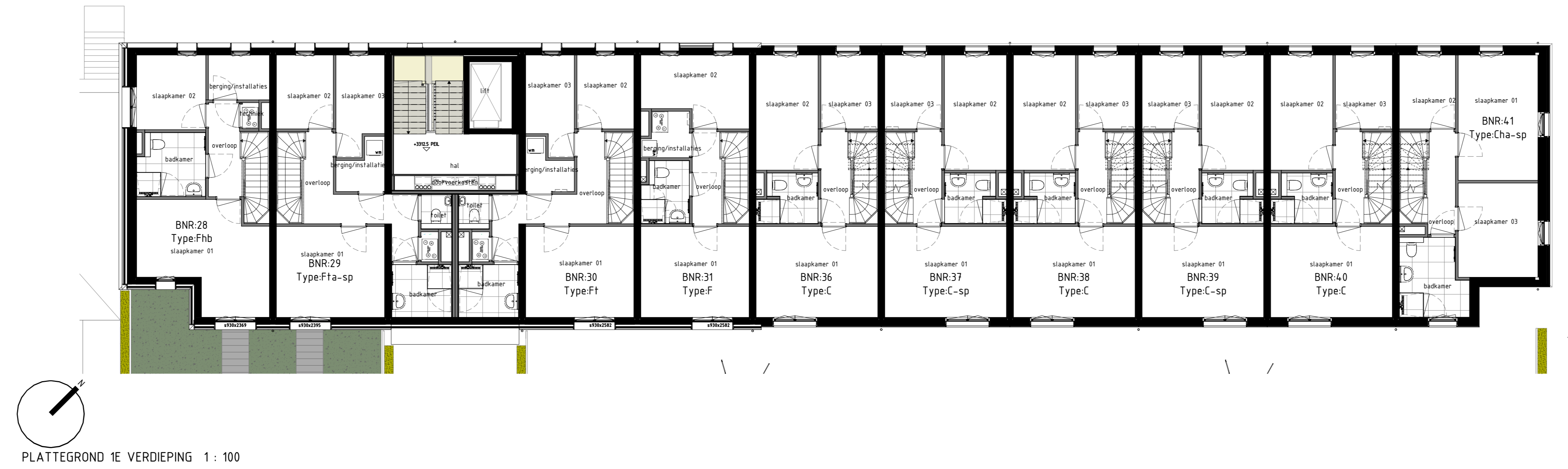
PLATTEGROND 1E VERDIEPING 1 : 100
