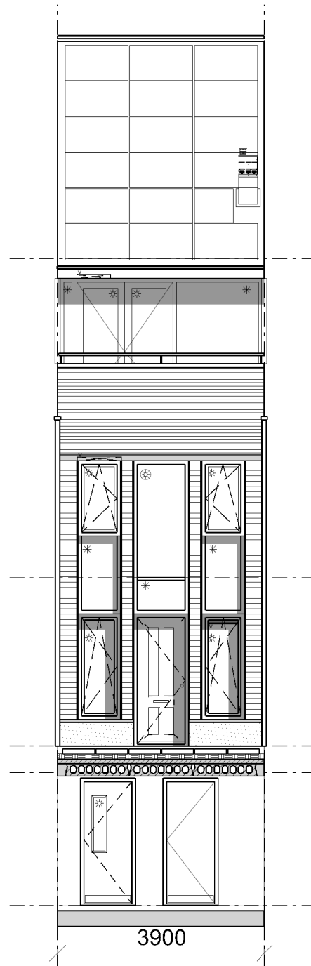
Gewel Straatzijde
