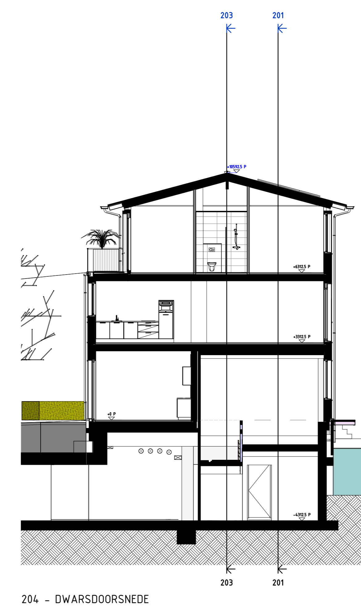
204 - DWARSDOORSNEDE
