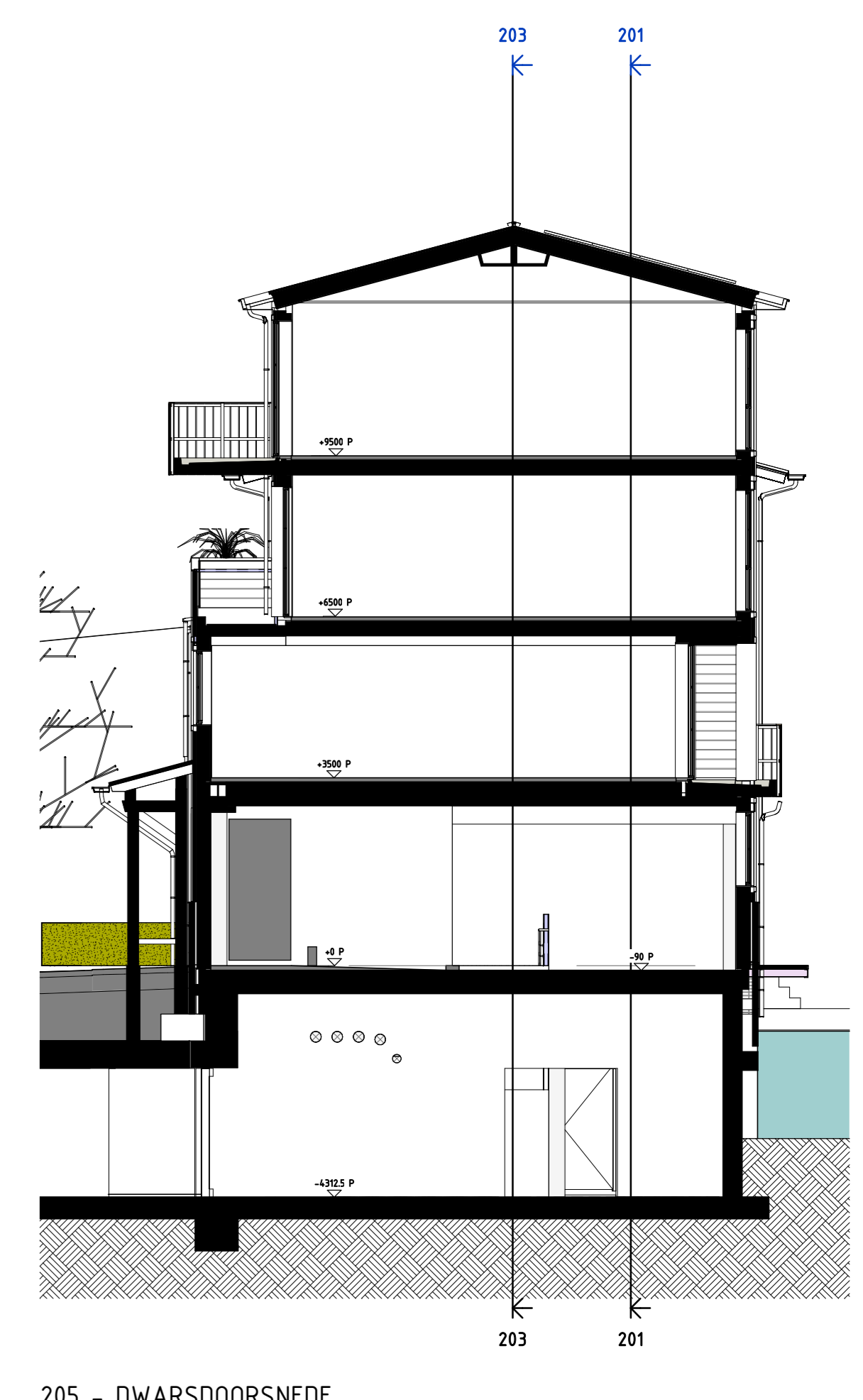
205 - DWARSDOORSNEDE
