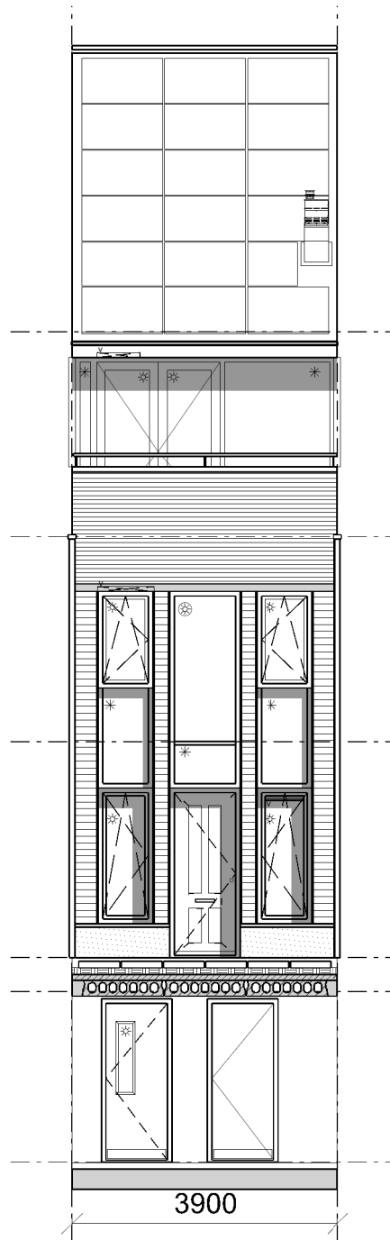
Gevel Straatzijde
