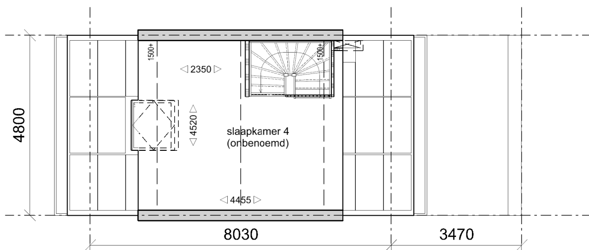
Verdieping 3
