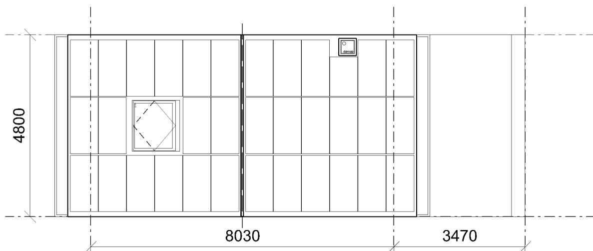
Dakaanzicht
