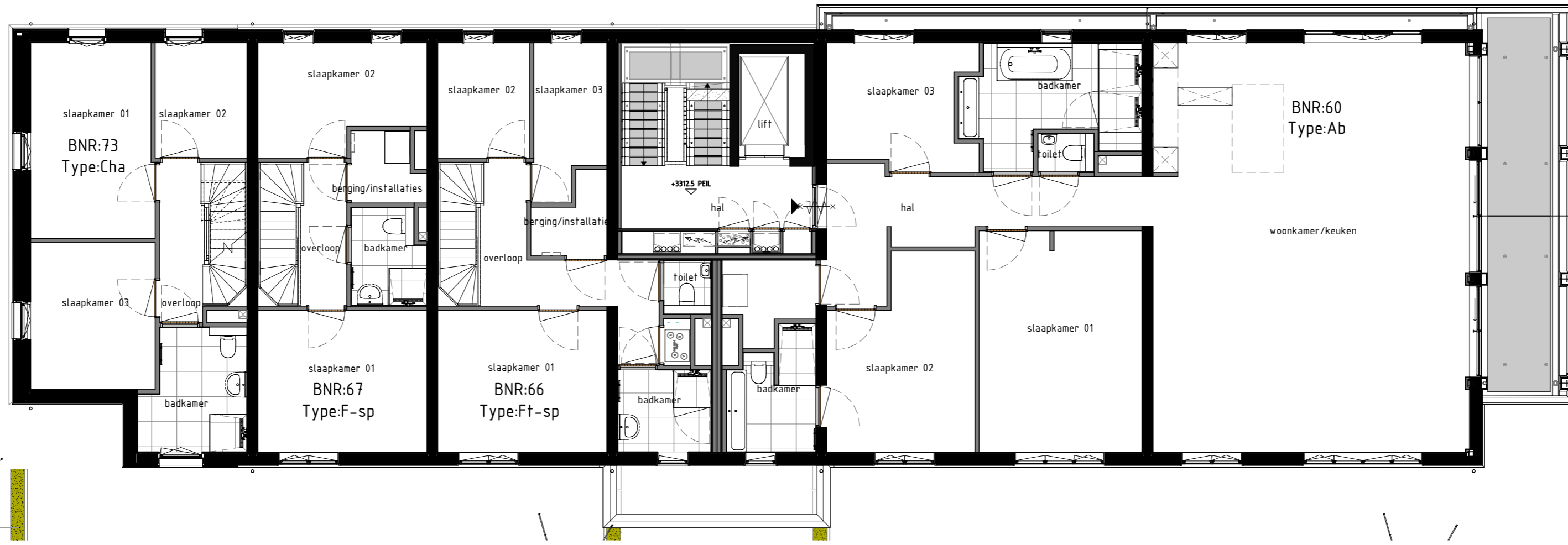
PLATTEGROND 1E VERDIEPING 1 : 100
