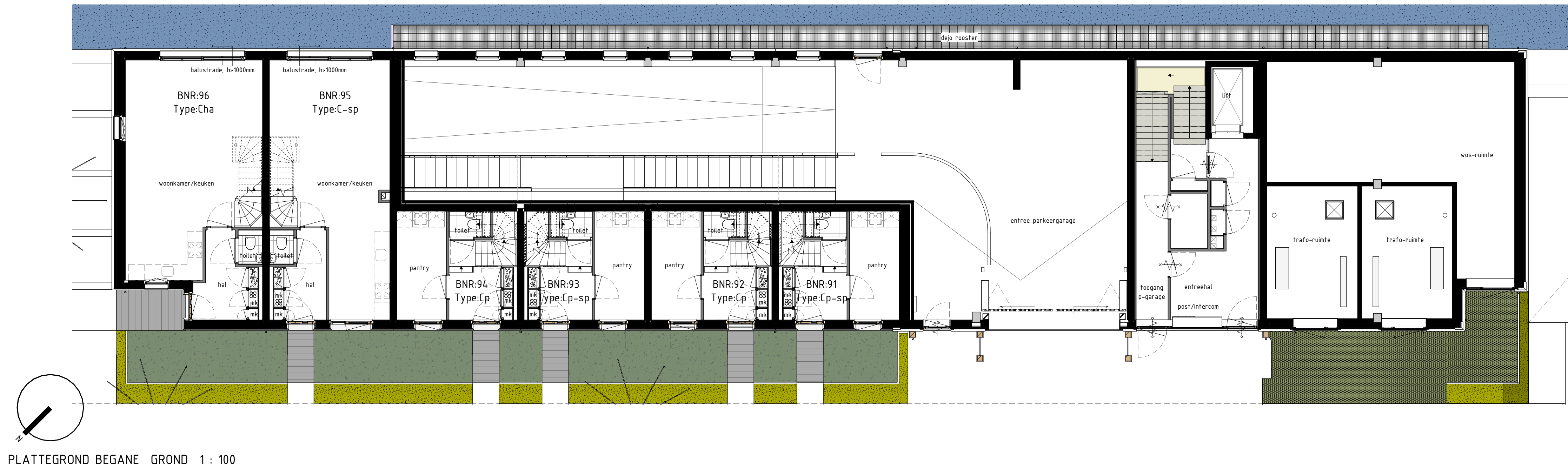
PLATTEGROND BEGANE GROND 1 : 100
