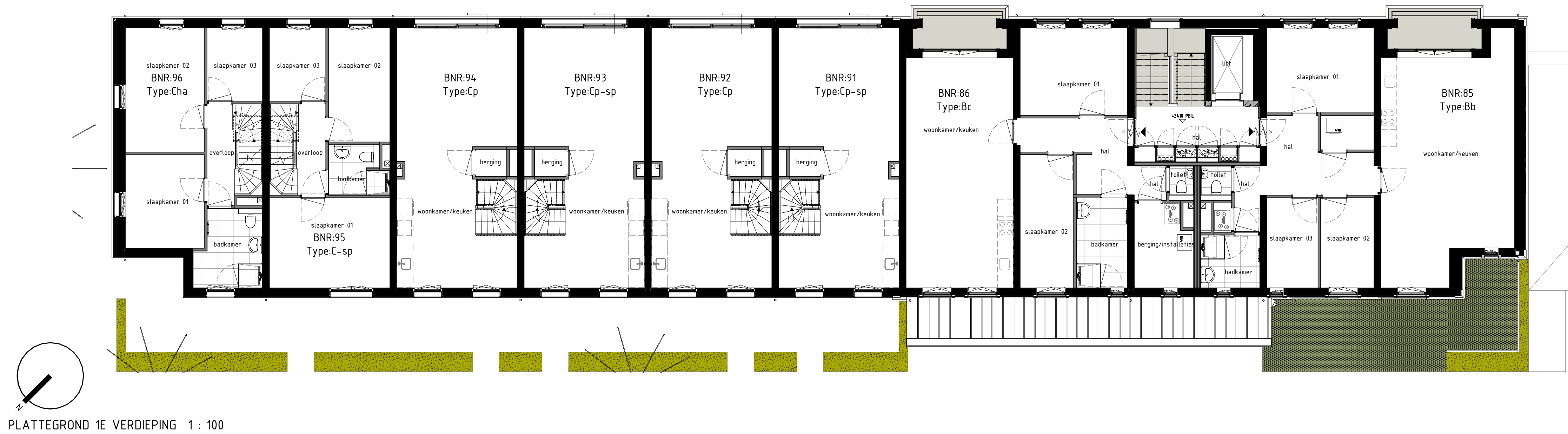
PLATTEGROND 1E VERDIEPING 1 : 100
