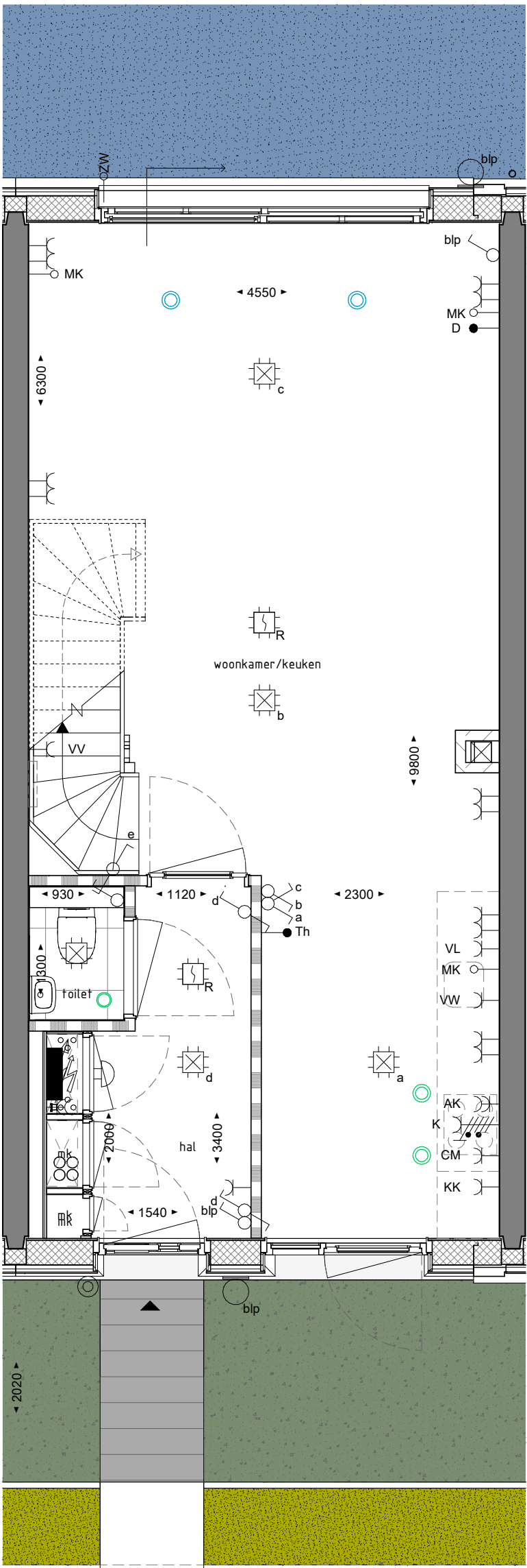
BEGANE GROND
