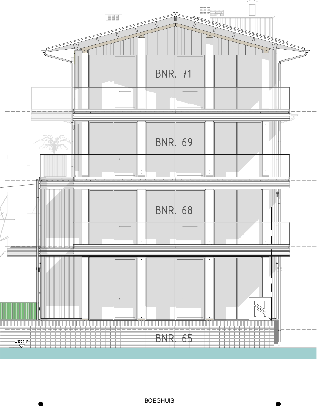
KOPGEVEL ZUID-WEST 1 : 100
