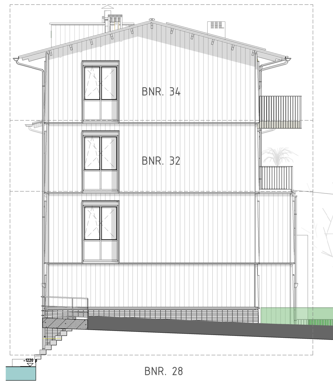
KOPGEVEL ZUID-WEST 1 : 100
