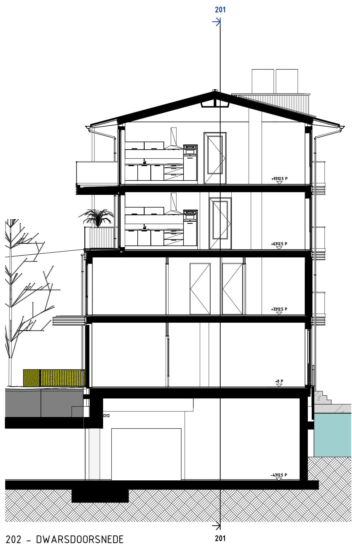
202 - DWARSDOORSNEDE
