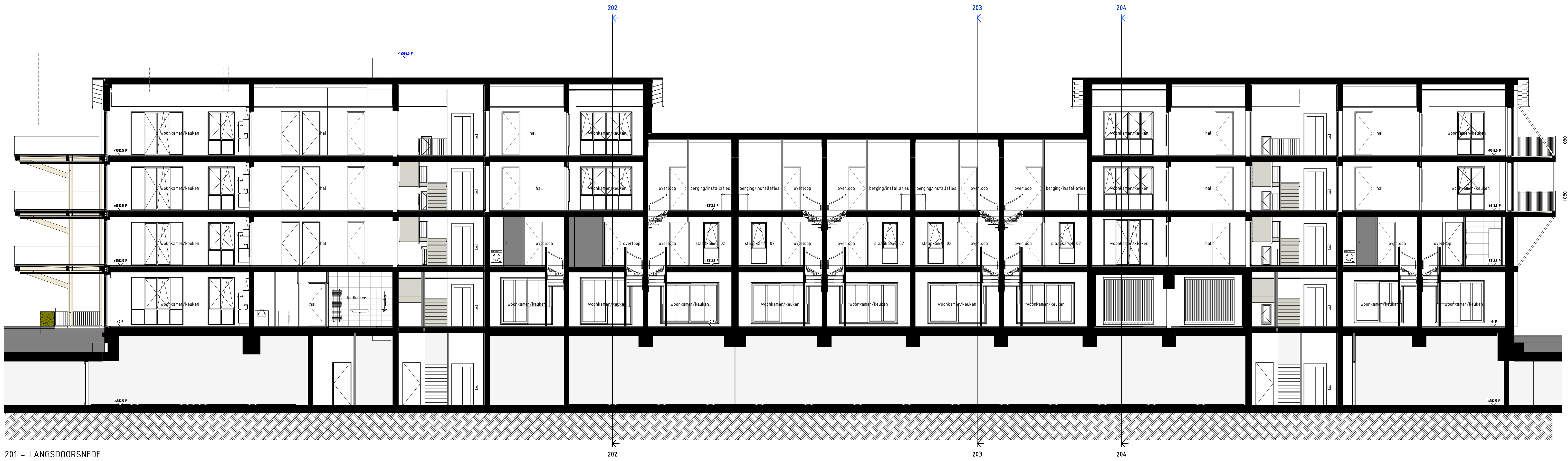
201 - LANGSDOORSNEDE
