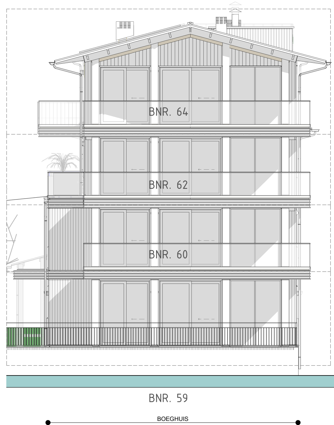
KOPGEVEL NOORD-OOST 1 : 100
