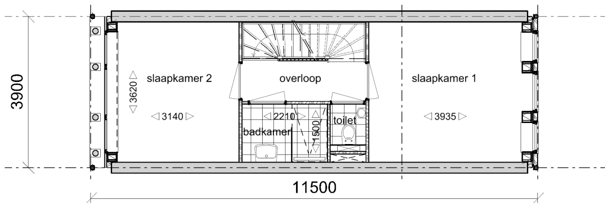
Verdieping 1
