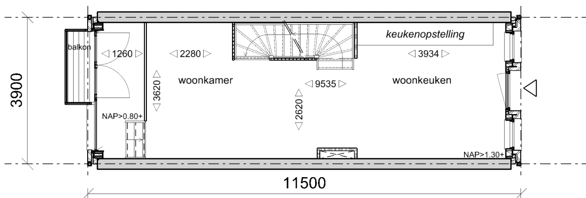
Begane grond
