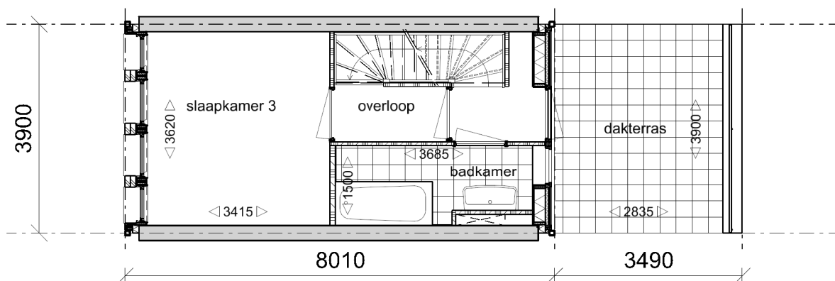
Verdieping 2
