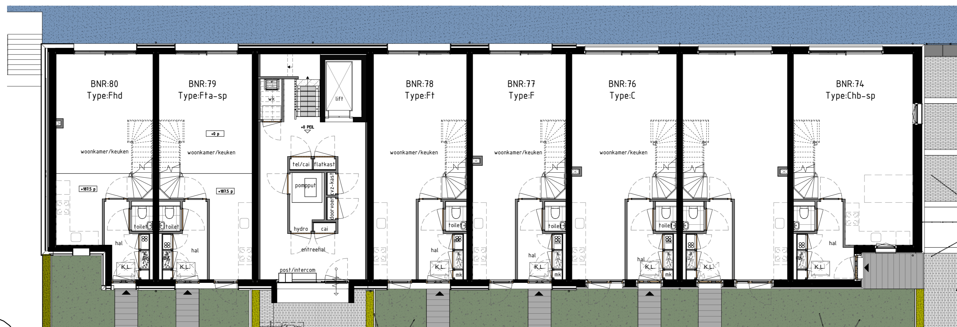
PLATTEGROND BEGANE GROND 1 : 100
