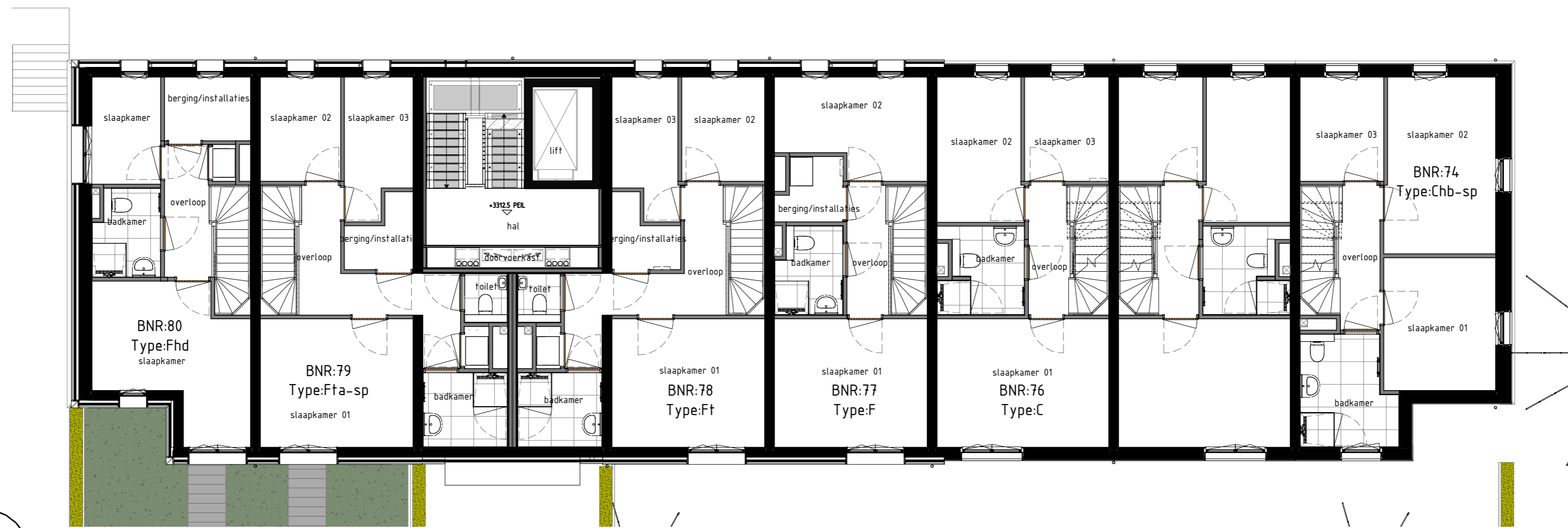
PLATTEGROND 1E VERDIEPING 1 : 100
