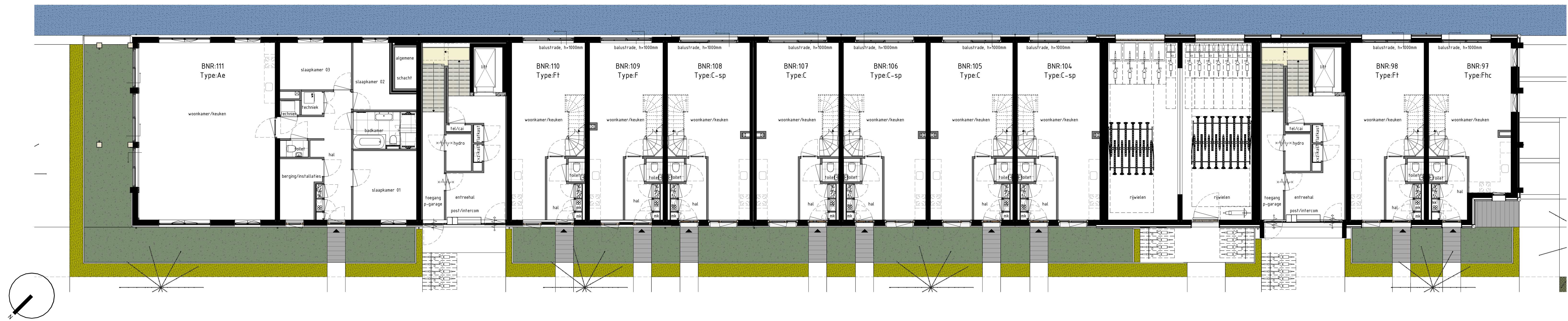
PLATTEGROND BEGANE GROND 1 : 100
